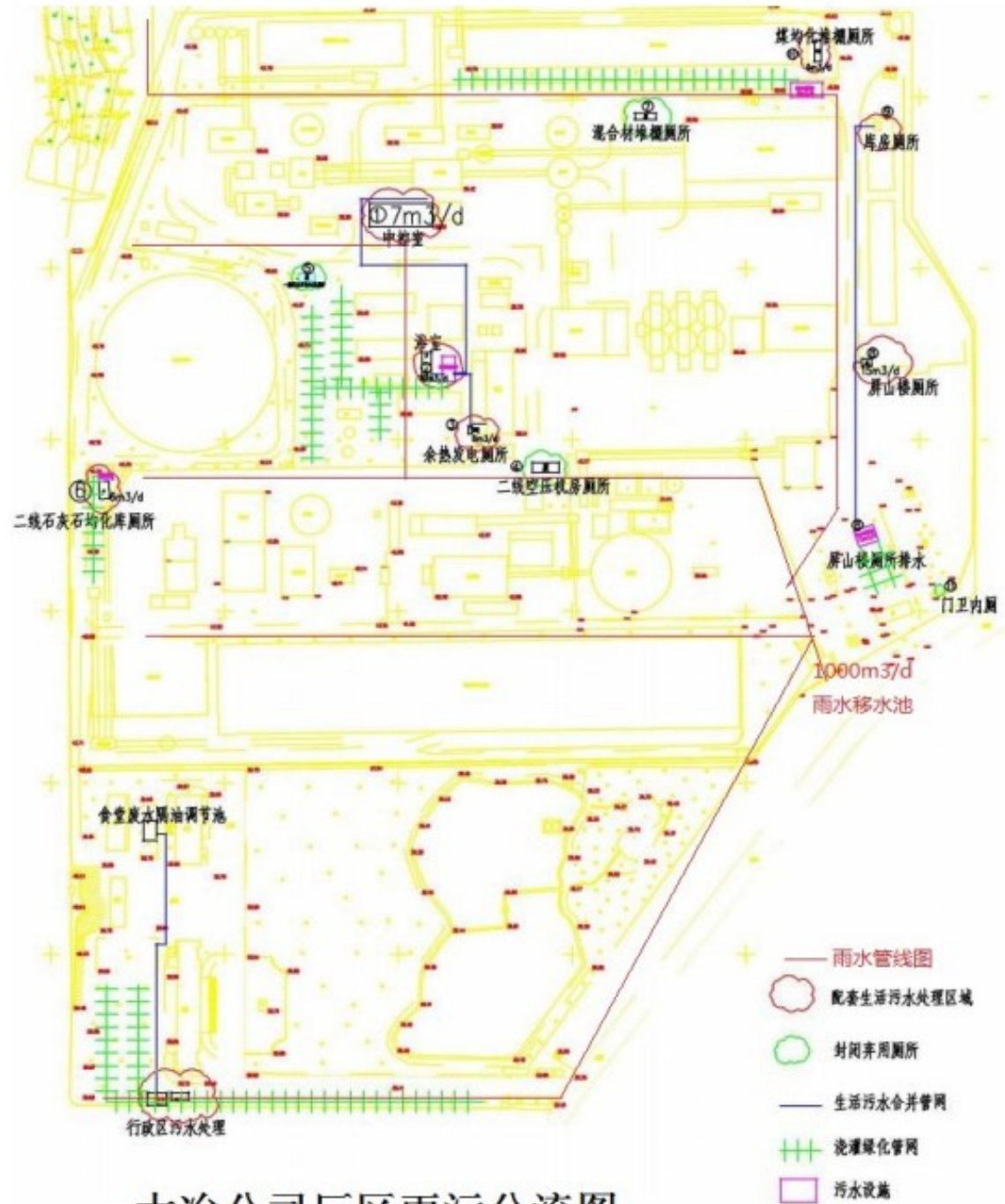
大冶公司厂区雨污分流图
